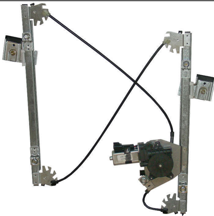
POWER WINDOW LEFT ALZACRISTALLI ELETTRICO SX
