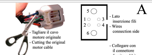
POWER WINDOW LEFT ALZACRISTALLI ELETTRICO SX
