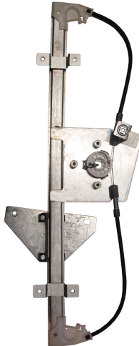
POWER WINDOW LEFT ALZACRISTALLI ELETTRICO SX
