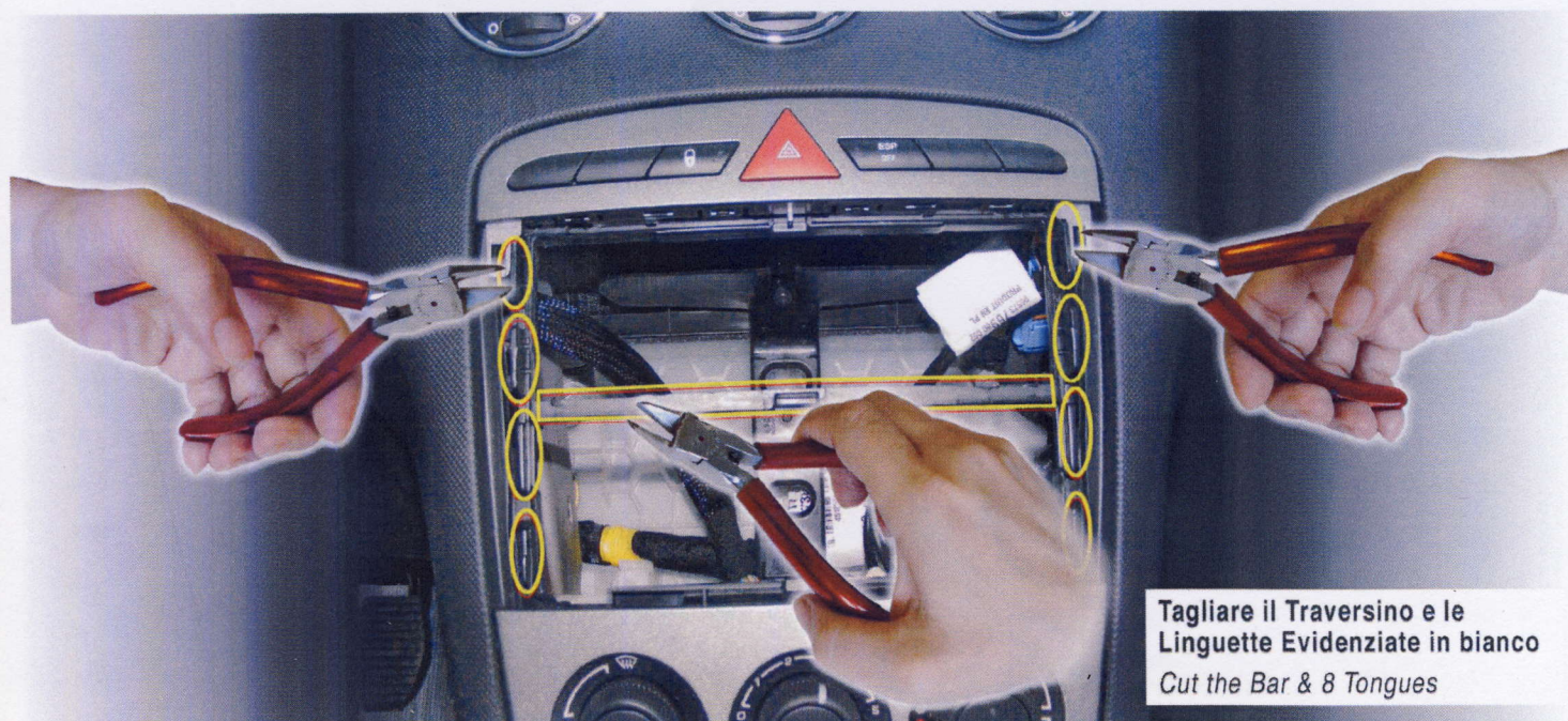
Tagliare il Traversino e le Linguette Evidenziate in bianco Cut the Bar & 8 Tongues
