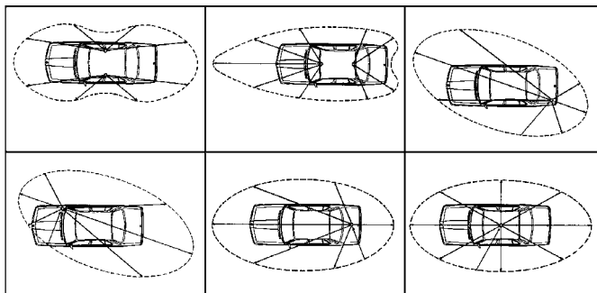
ANTENNEN-DIAGRAMM
