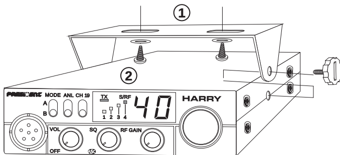
BEFESTIGUNG DES MONTAGEBÜGELS
