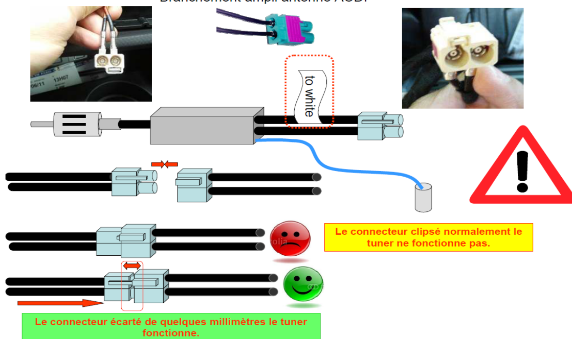
Branchement ampli antenne AUDI
