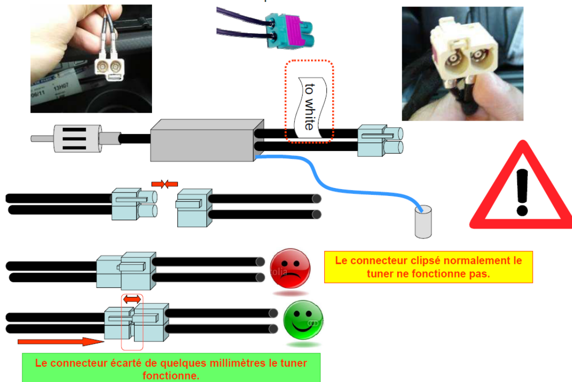
Branchement ampli antenne AUDI
