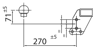
26029/VM
