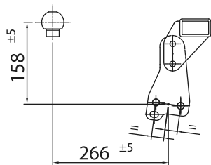
26029/C - 26029/F
