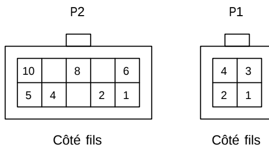
Disposition câblage pour interface RG8
