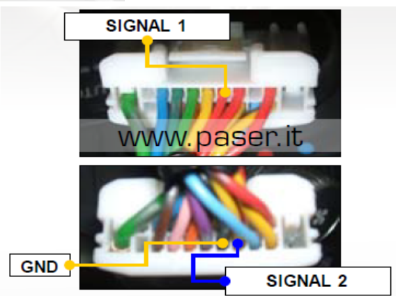
Vue arrière connecteur du véhicule côté fil
