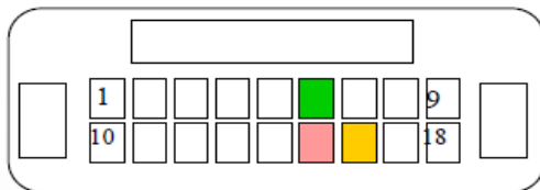
Vue arrière connecteur du véhicule côté fil
