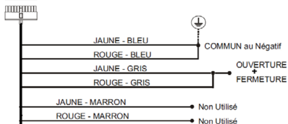
SCHÉMA N°2
