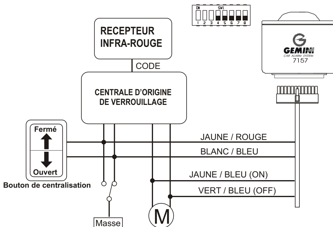
Schéma avec transmission codifié du récepteur, avec bouton de commande libre au repos
