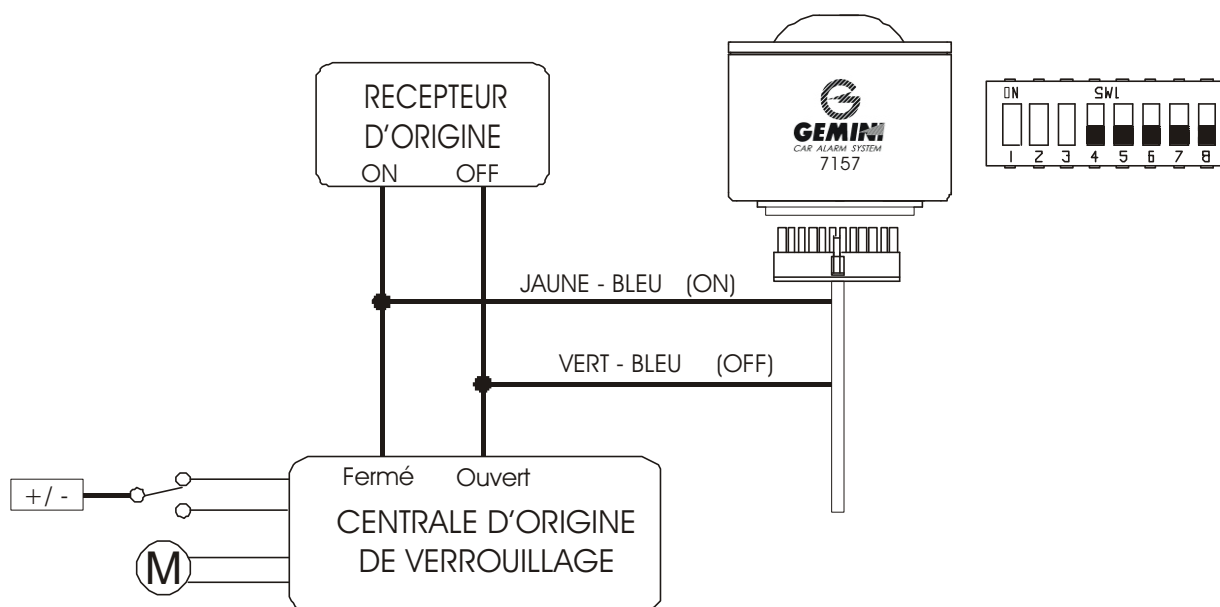
Schéma pour commande Positive
