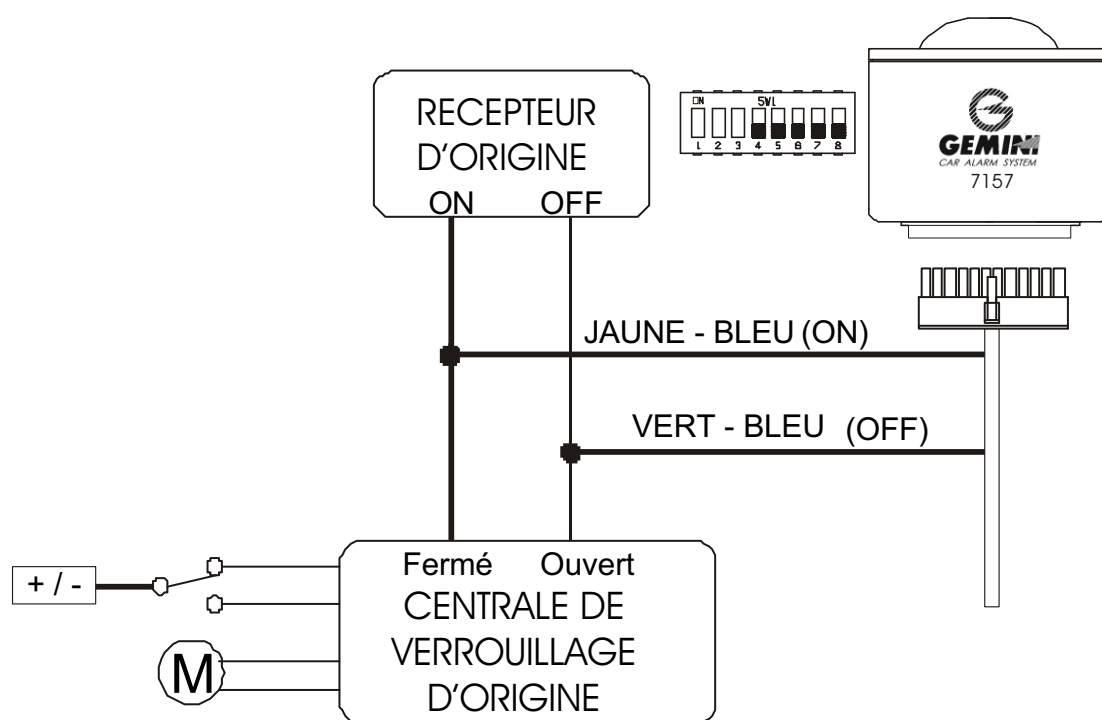
Schema pour commande Positive
