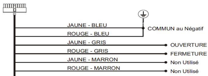
SCHÉMA N°2
