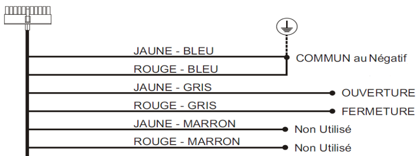
SCHÉMA N°2
